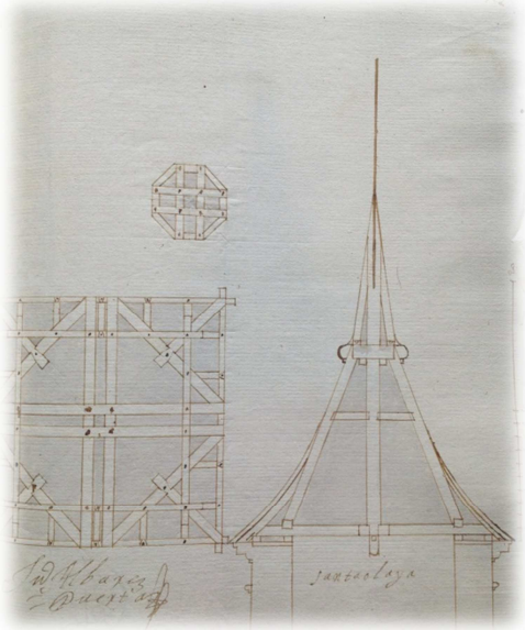
Plano de la estructura de la cubierta - 1721
